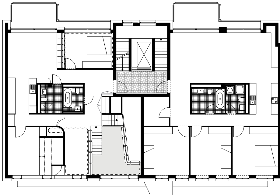
4. Etage
