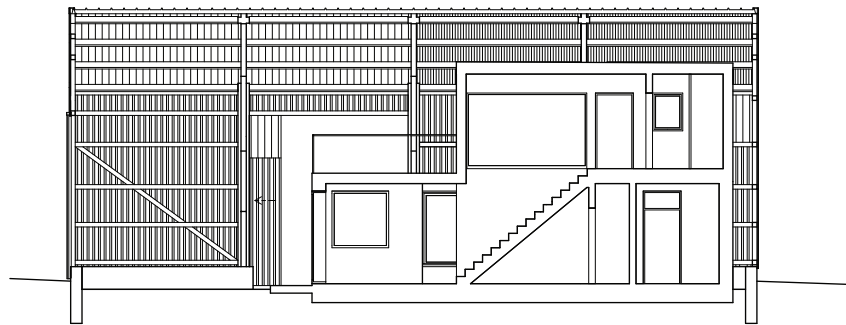
Längsschnitt
