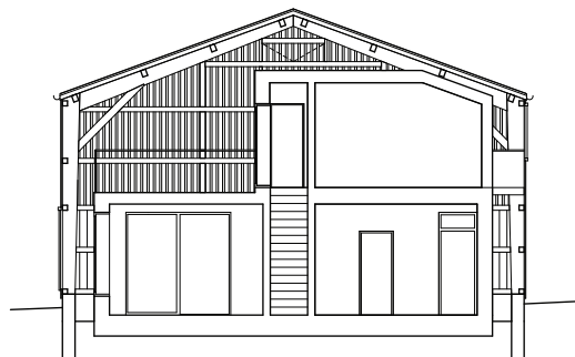
Querschnitt
