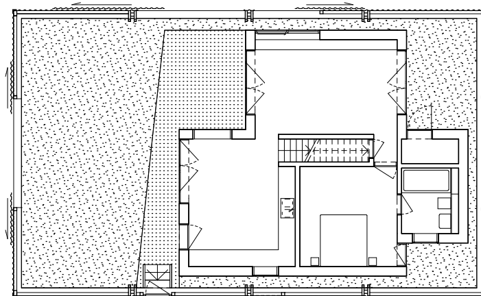
Grundriss E6
