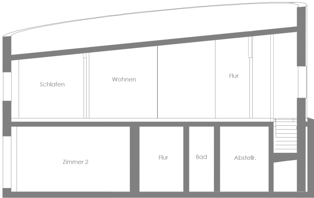
Schnitt A-A
