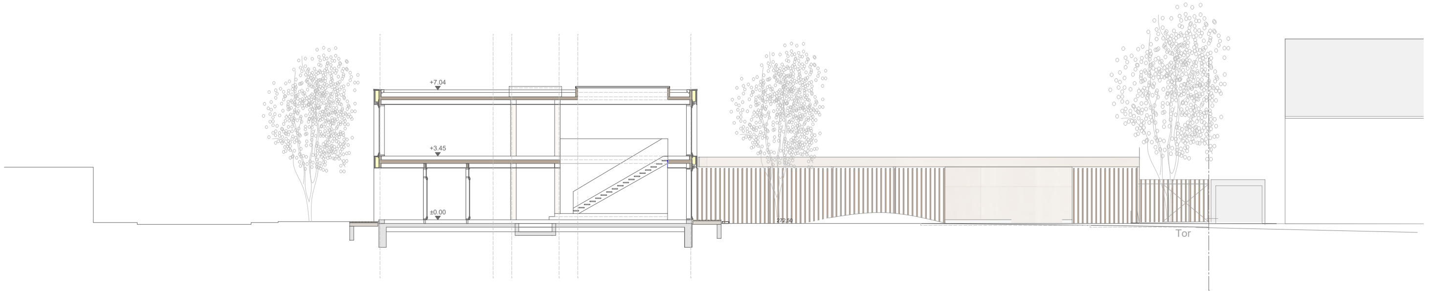
Querschnitt
