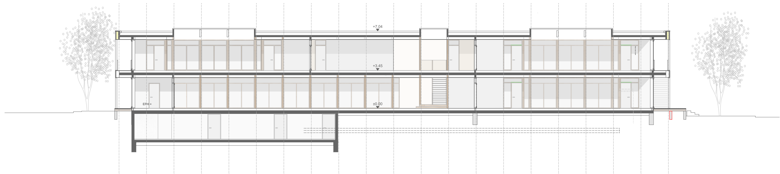
Längsschnitt
