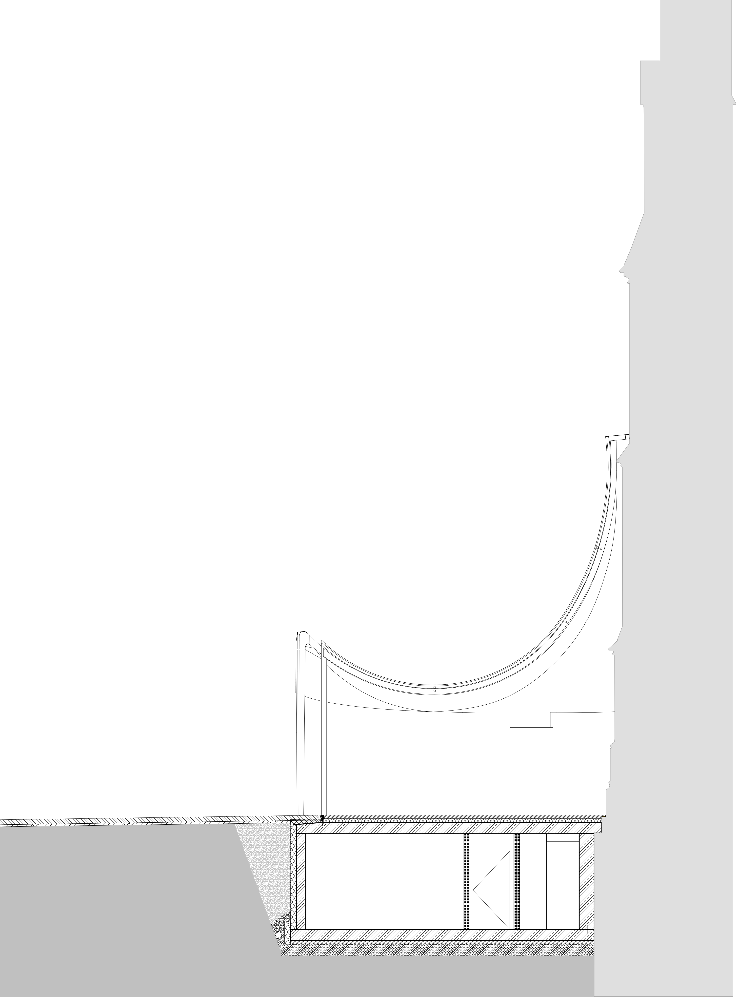
Schnitt 1-1 1:50
