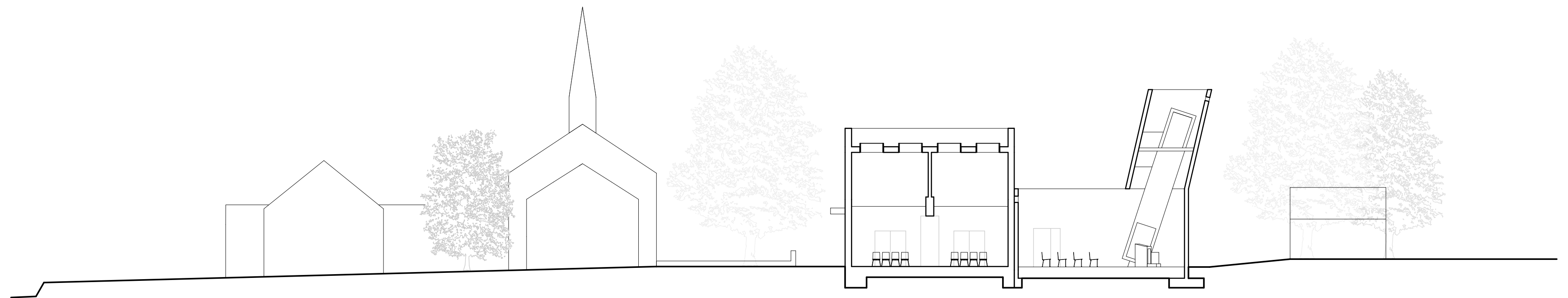
SCHNITT LANG
