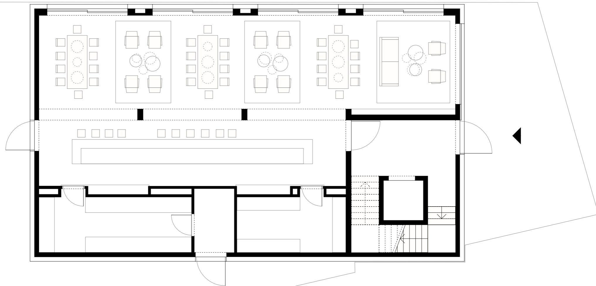
Grundriss Erdgeschoss
