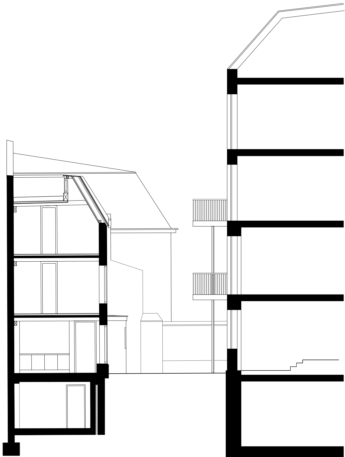
QUERSCHNITT
