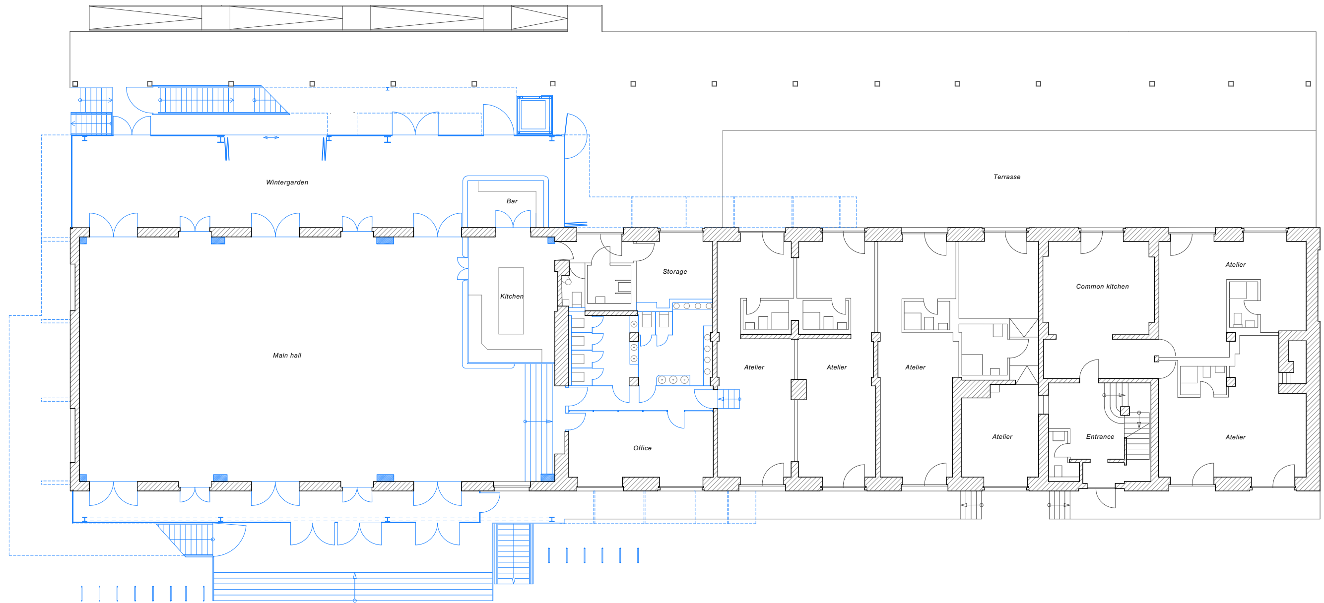
Grundriss Erdgeschoss
