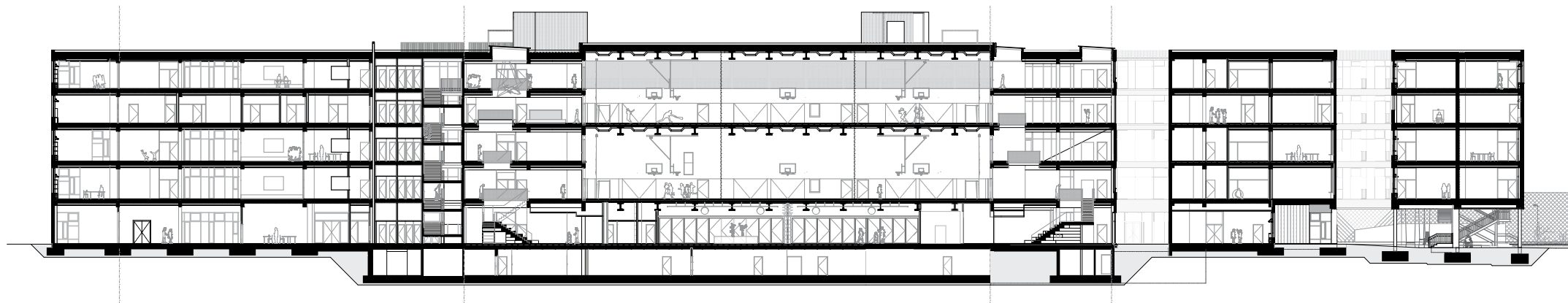
SCHNITT A-A
