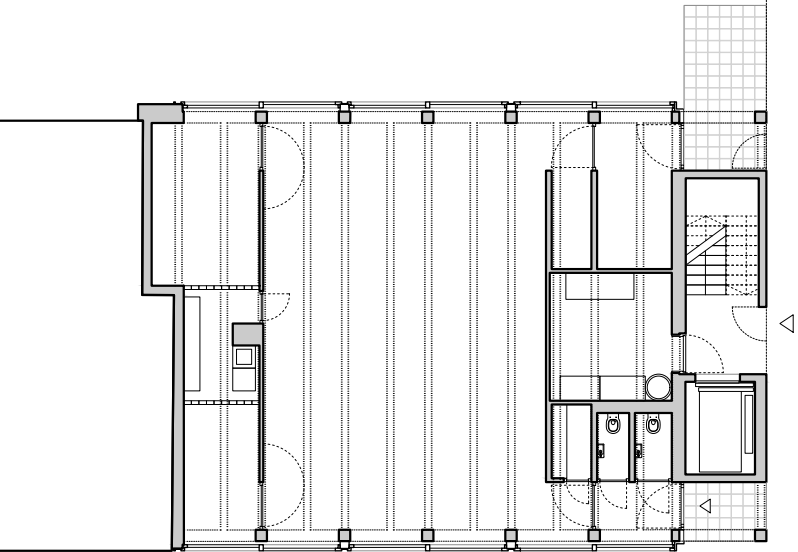
Erdgeschoss M 1:200
